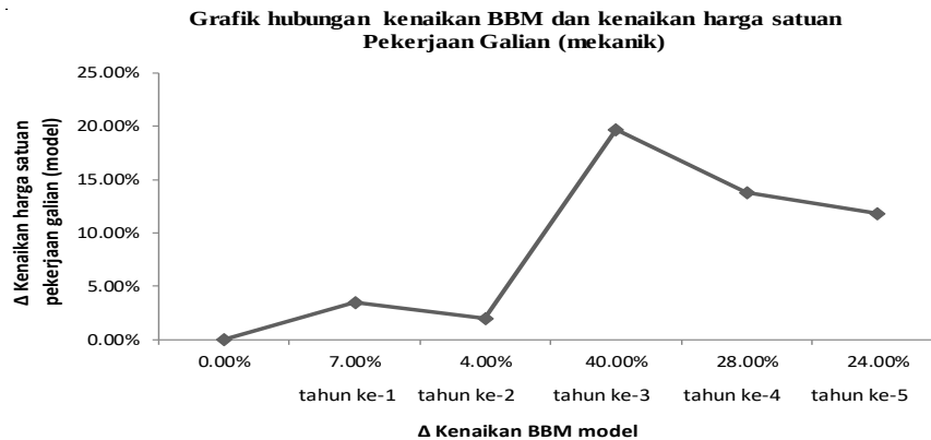
Gambar 3 Grafik hubungan kenaikan BBM dan kenaikan harga satuan Pekerjaan Galian Analisis Sensitivitas Metoda Regresi
