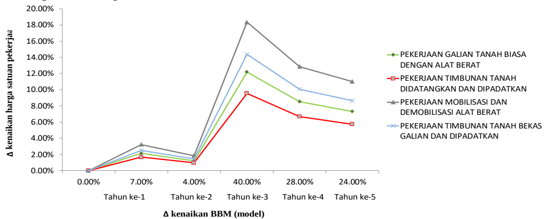
Gambar 5 rekap grafik hubungan kenaikan BBM dan kenaikan harga satuan pekerjaan pada proyek SDA
