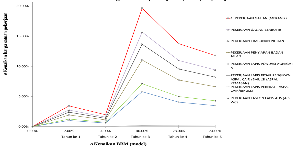
Gambar 4 Rekap grafik hubungan kenaikan BBM dan kenaikan harga satuan pekerjaan pada proyek jalan.
